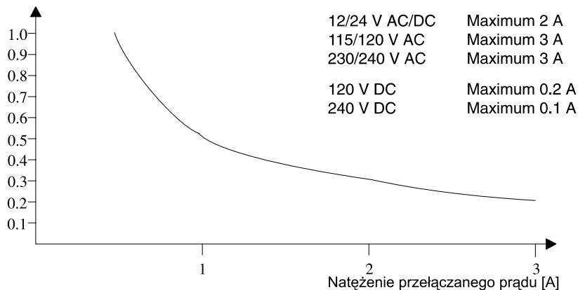
Rys. B. Trwałość łączeniowa i żywotność styków dla wysokich obciążeń indukcyjnych wg IEC 947-5-1 DC 13/AC 15 (styczniki, elektromagnesy, silniki)
