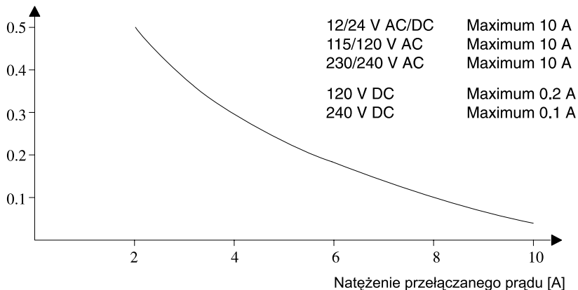
Rys. A. Trwałość łączeniowa i żywotność styków dla obciążeń rezystancyjnych (ogrzewanie)
